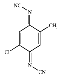
MeCl-DCNQI
