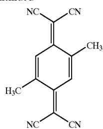
TCNQ-(CH 3 ) 2
