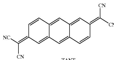
TANT
