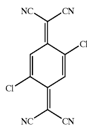
TCNQ-Cl 2
