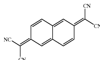
TNAP
