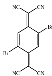
TCNQ-Br 2
