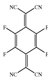
TCNQ-F 4
